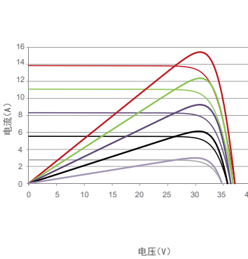
电流电压及功率电压曲线(405W)
