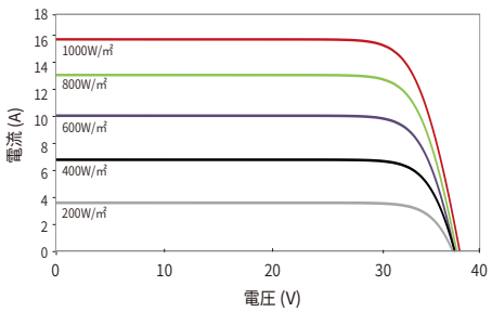
電流-電圧曲線 (51QL6-DB 505W)
