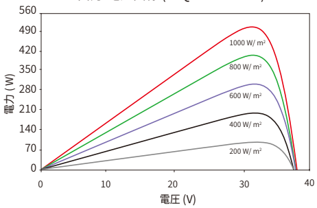
出力-電圧曲線 (51QL6-DB 505W)
