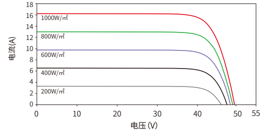
电流-电压曲线 66HL4M-BDV 635W
