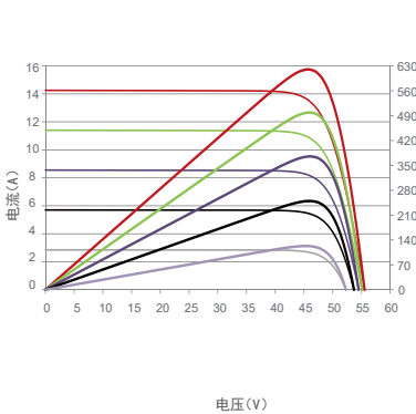
电流电压及功率电压曲线(620W)
