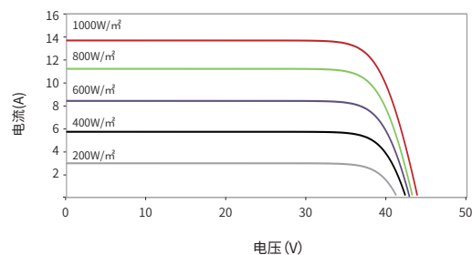
电流-电压曲线 60HL4-(V) 480W
