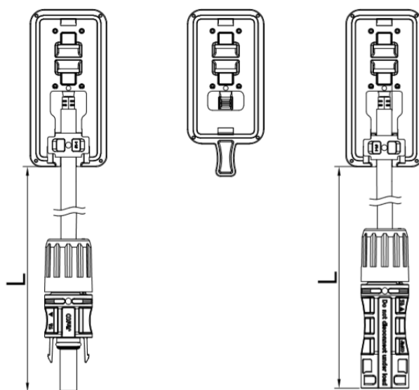
图13 (2) 半片/透明背板双面组件接线盒
