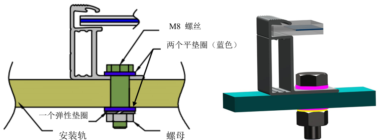
图2 螺栓安装示意图
