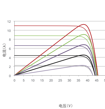
电流电压及功率电压曲线(355W)
