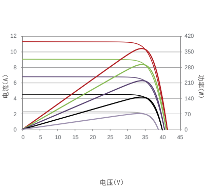
电流电压及功率电压曲线(365W)
