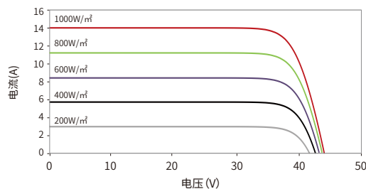
电流-电压曲线 60HL4-(V) 490W
