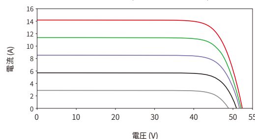
電流-電圧曲線 (72HL4-BDV 590W)
