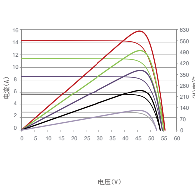
电流电压及功率电压曲线(620W)
